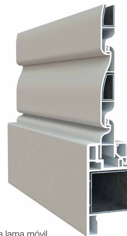
Detalle lama móvil
